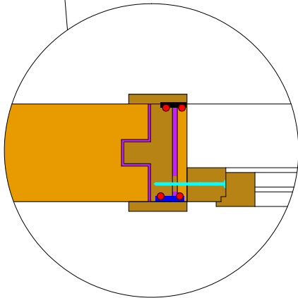
Systemzeichnung ohne Maßstab
